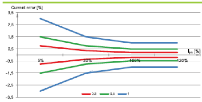
a) classes 0.2; 0.5; 1
